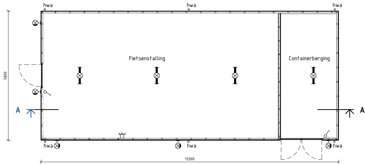
PLATTEGROND
