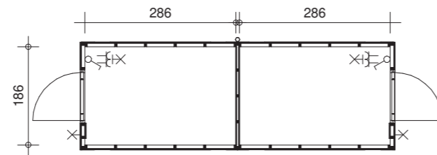
Dubbele berging
