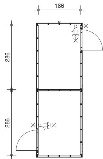
Dubbele berging
